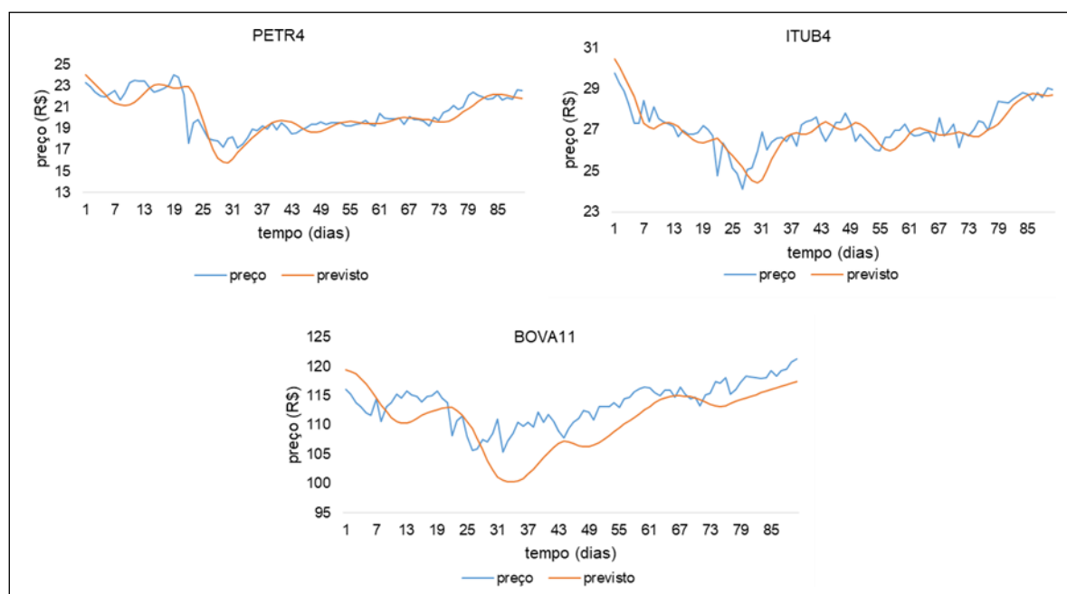
Figura 4: Valores reais e preditos das ações para o modelo LSTM.
