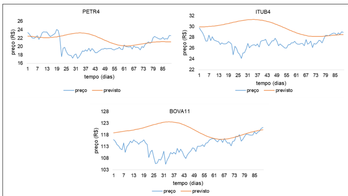
Figura 3: Valores reais e preditos das ações para o modelo PROPHET
