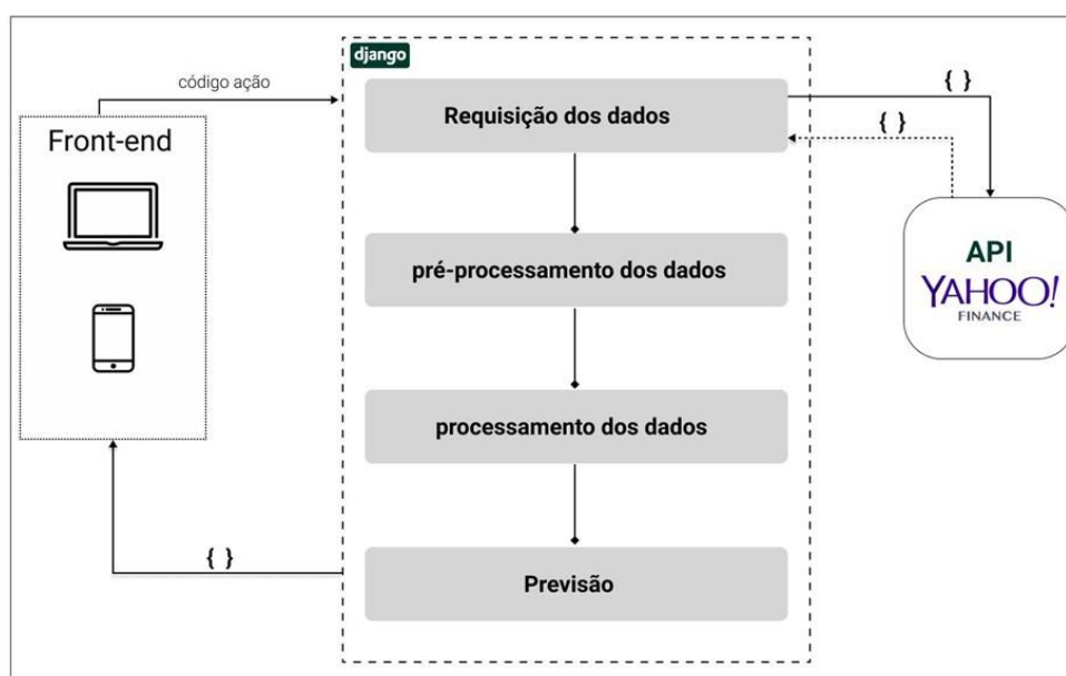
Figura 5: Arquitetura do protótipo (the seer)
