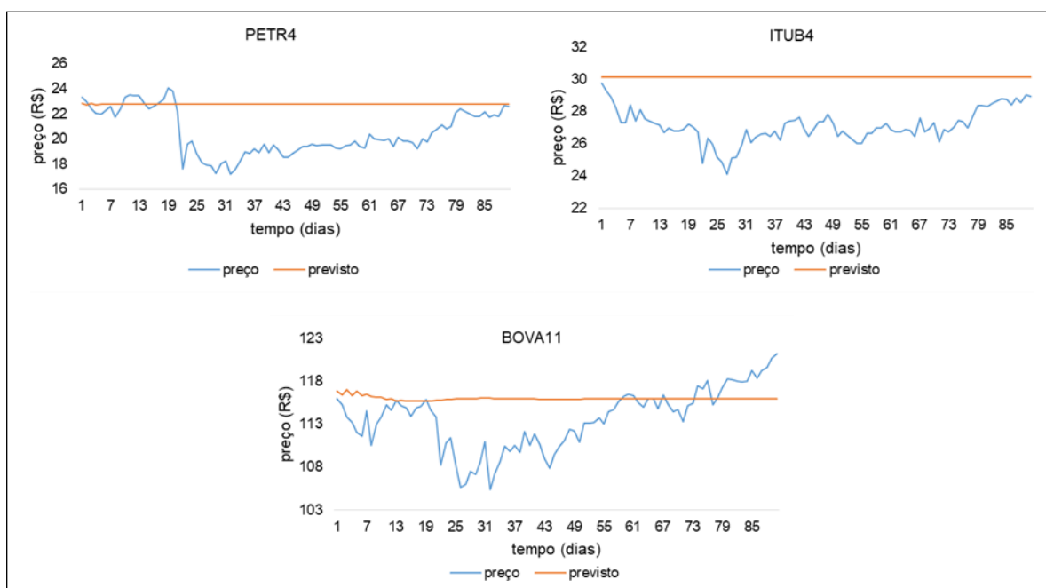
Figura 2: Valores reais e preditos das ações para o modelo ARIMA.
