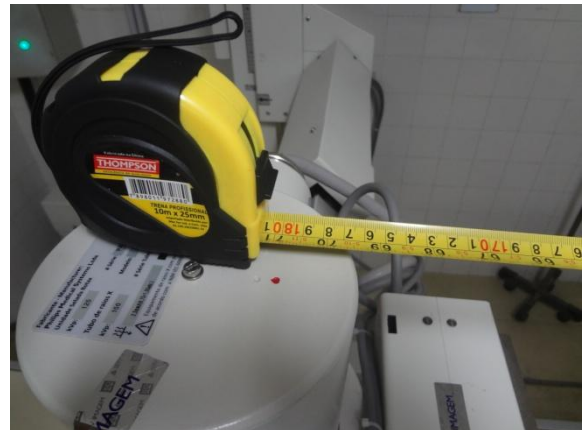
Figura 3 – Ajuste da distancia entre o bucky vertical e o ponto focal em 1,80 metros.
