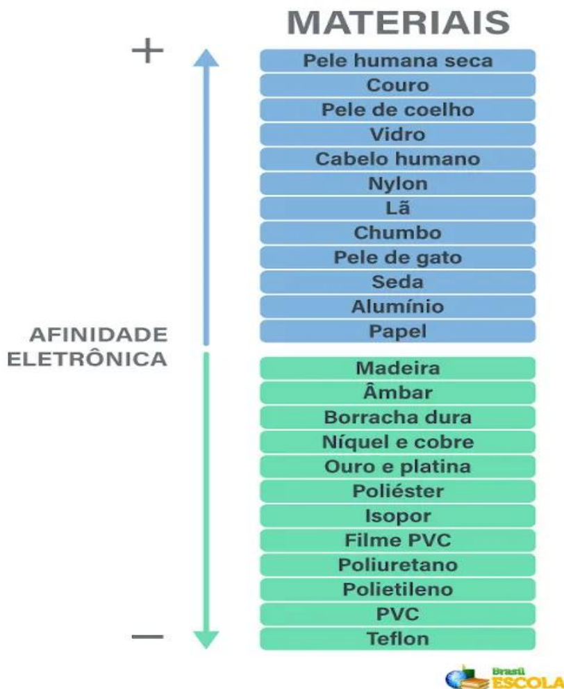
Figura 5: Série triboelétrica
