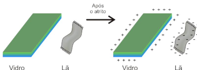
Figura 6 - Ilustração do antes e depois do processo de eletrização
