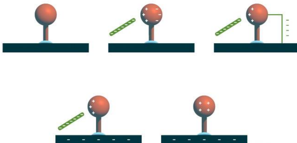
Figura 10 - Processo de eletrização por indução
