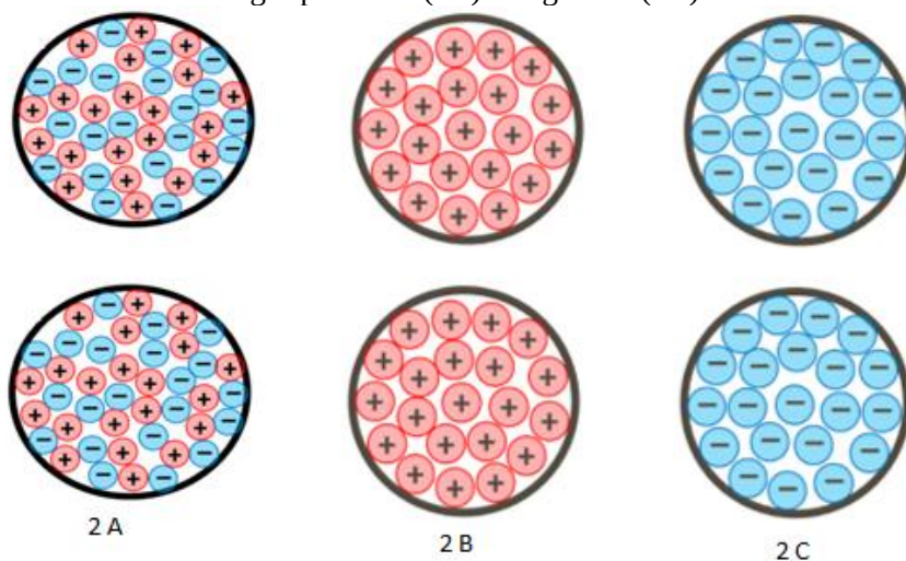
Figura 2 - Representação esquemática de carga elétrica em equilíbrio (2A) e em excesso de cargas positivas (2B) e negativas (2C)
