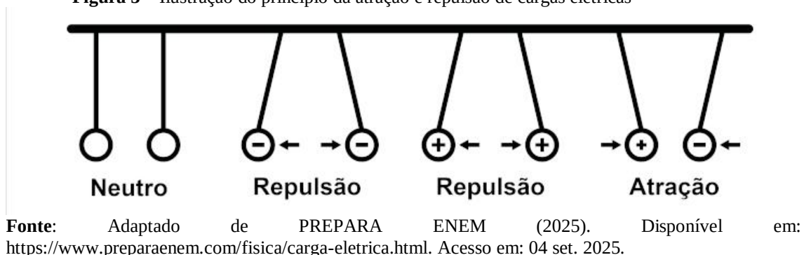
Figura 3 – Ilustração do princípio da atração e repulsão de cargas elétricas
