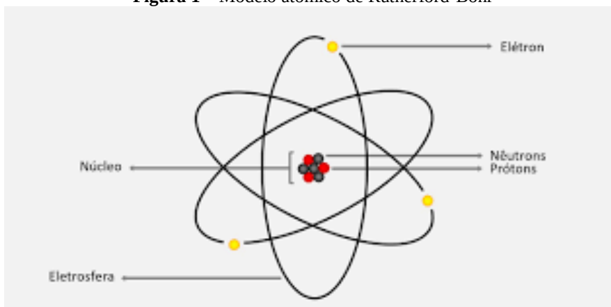
Figura 1 – Modelo atômico de Rutherford-Bohr
