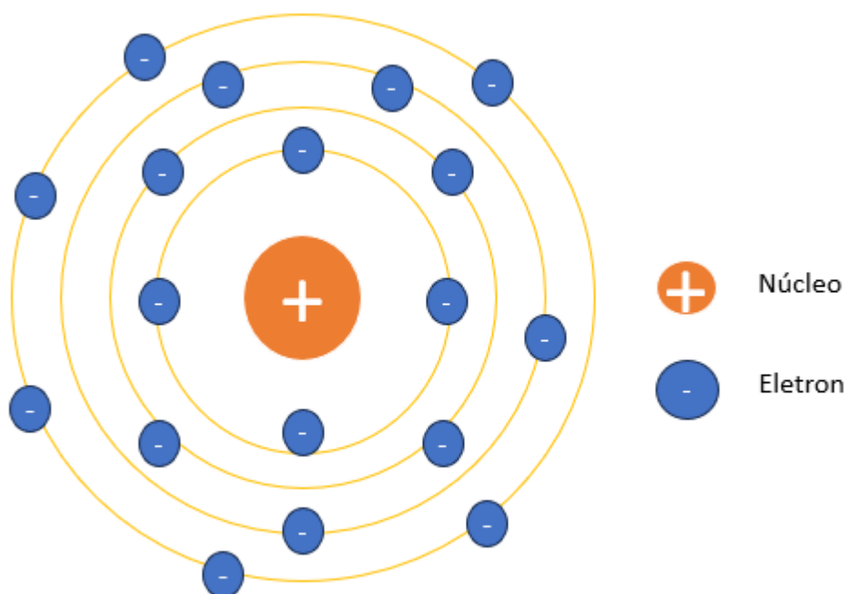
Figura 3: Modelo de Rutherford-Bohr, camadas eletrônicas e elétrons, processos de eletrização.
