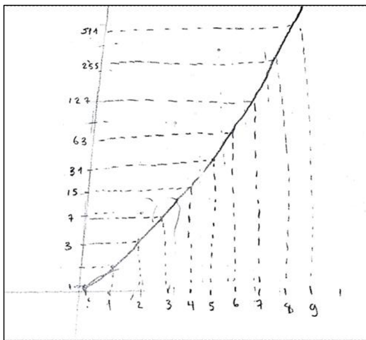
Figura 37 – Gráfico do modelo T(n) = 2^n - 1 .
