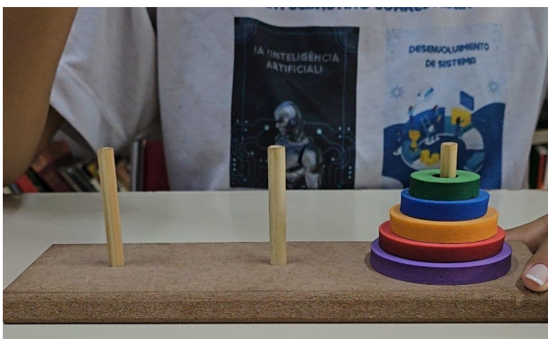
Figura 35 - Torre de Hanói com cinco discos
