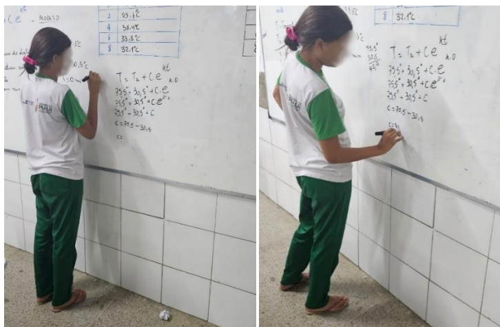
Figura 50 - Aplicação da Lei de Resfriamento de Newton
