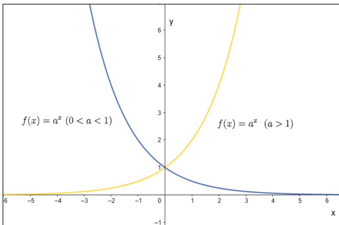
Figura 2 – Gráfico da função f(x) = a^x , com a > 1 (crescente) e 0 < a < 1 (decrecente)
