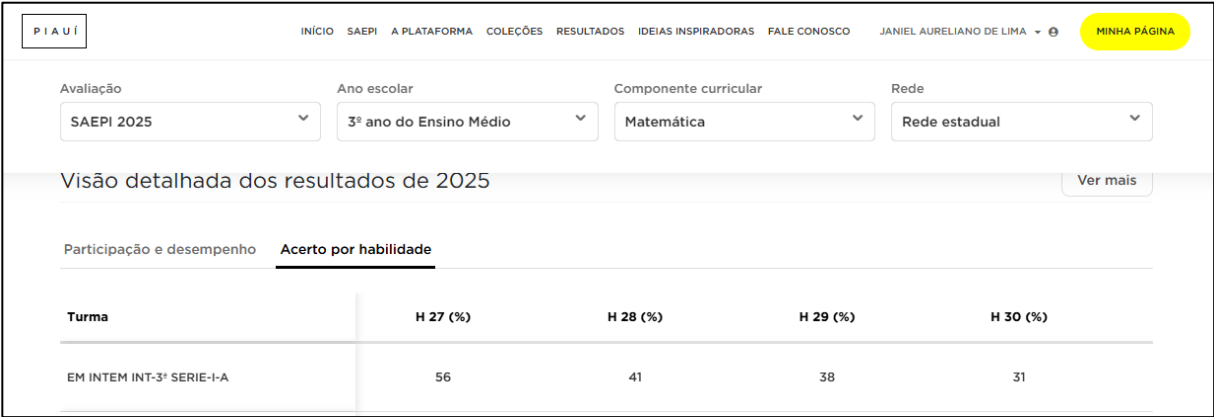
Figura 64 - Resultado SAEPI 2025
