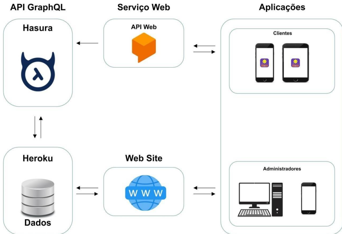
Figura 5. Apresenta a arquitetura da aplicação.
